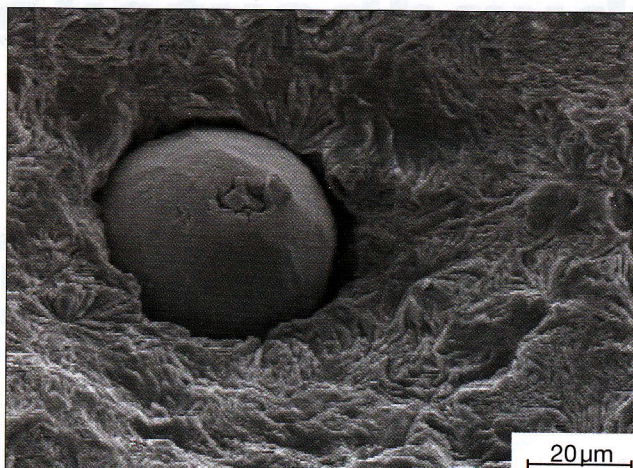
Abb. 2: Chemisch geätzter Anschlag eines thermisch leitfähig modifizierten Polyoxymethylen (POM). Mischungsverhältnis: POM + 60% Vol.-% Kupfer (Cu). Rasterelektronenmikroskop (REM) – Betrachtung der Kunststoffstruktur und der Füllstoff-Matrix-Anbindung.
